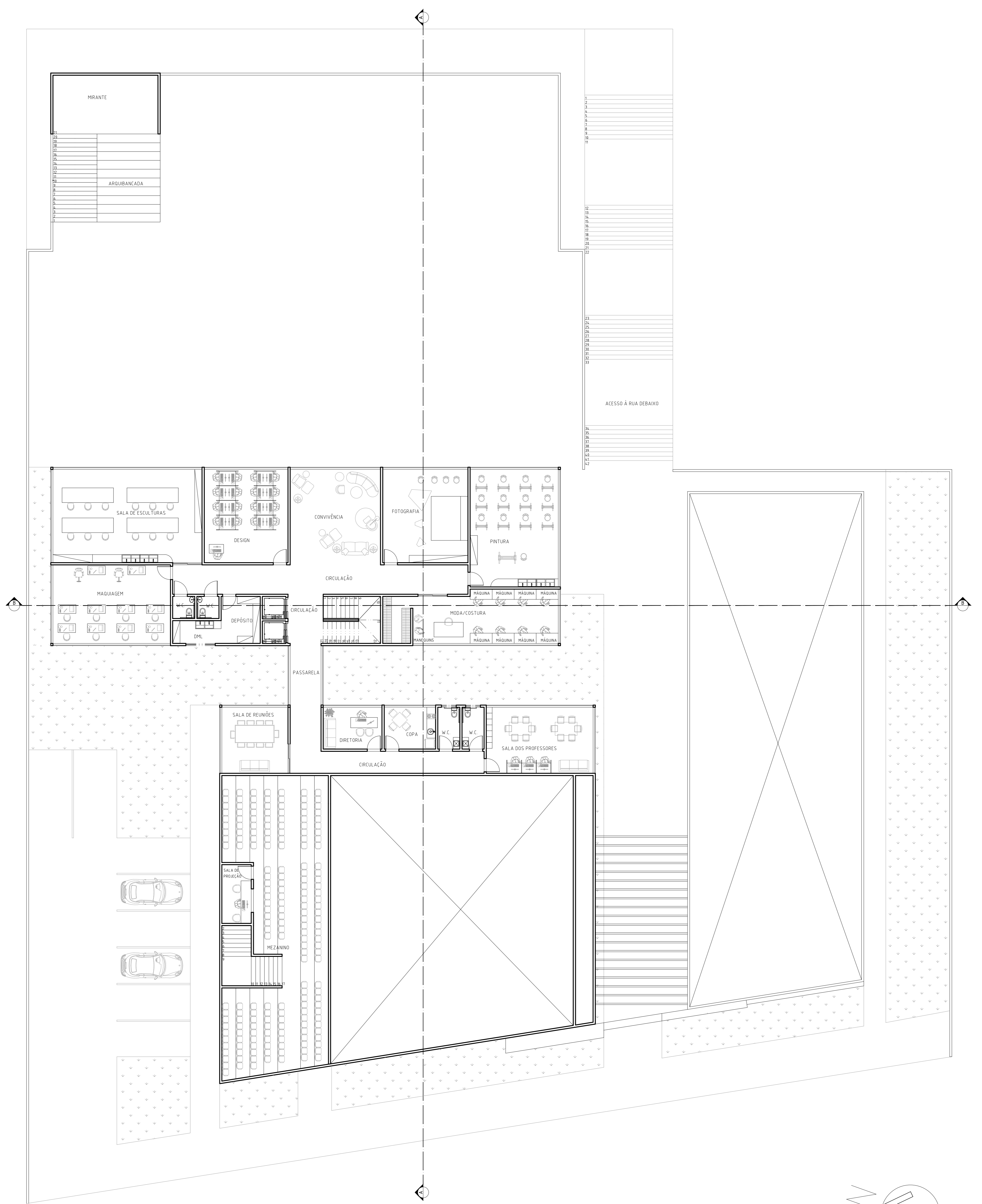
PLANTA LAYOUT 3º PAV ESCALA 1/25
