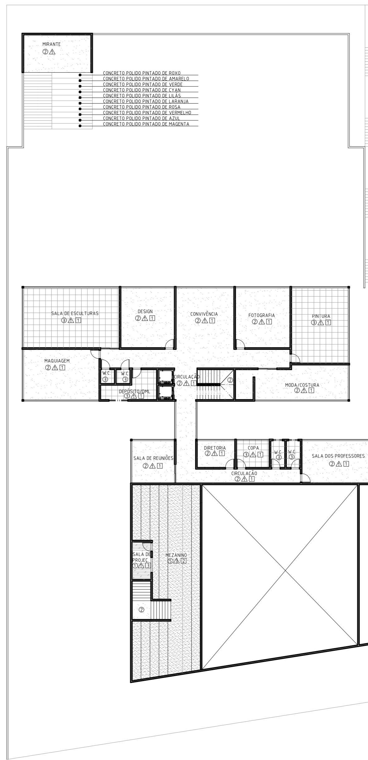
PLANTA PAGINAÇÃO DE PISO 3º PAV ESCALA 1/250
