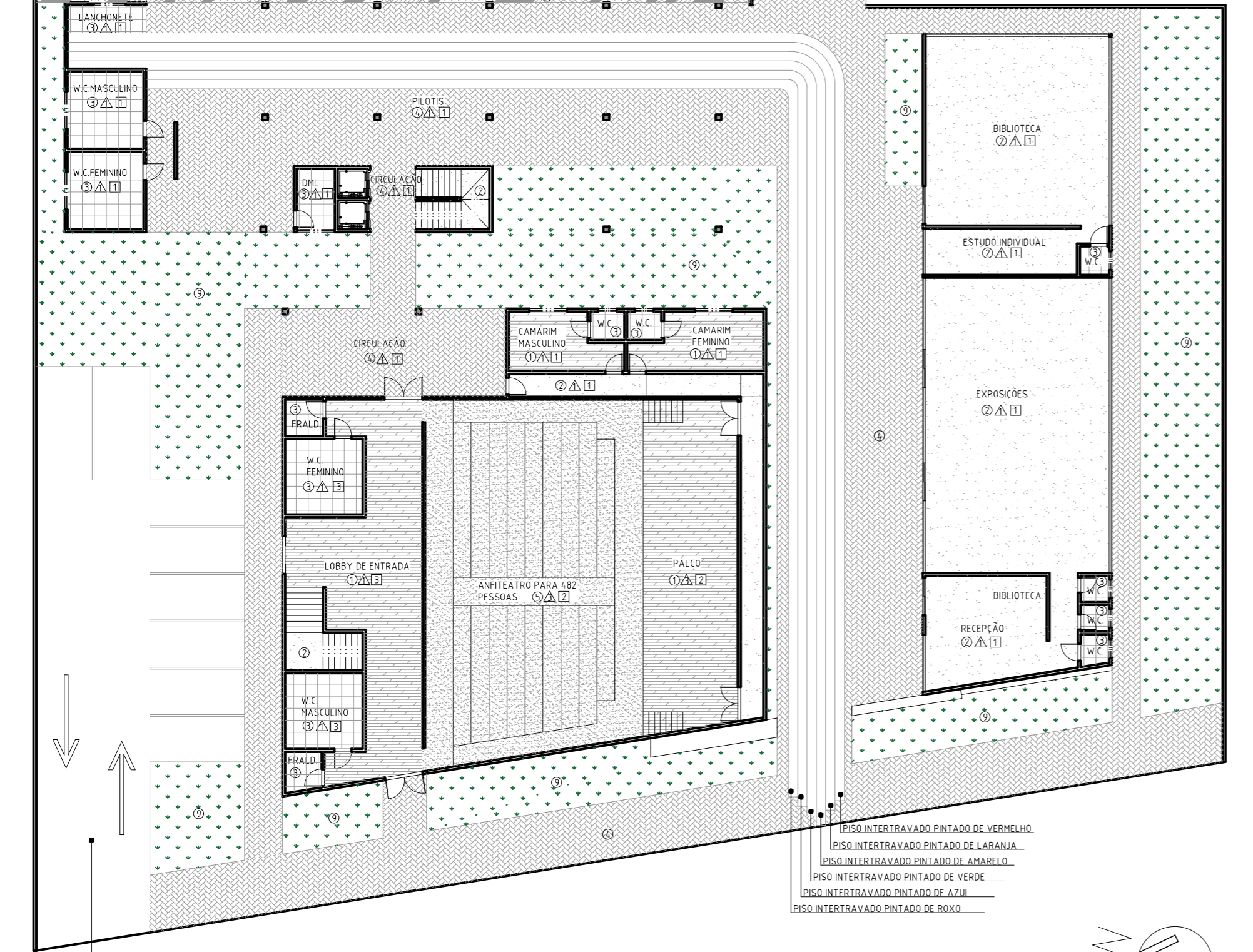
PLANTA PAGINAÇÃO DE PISO 2º PAV ESCALA 1/250
