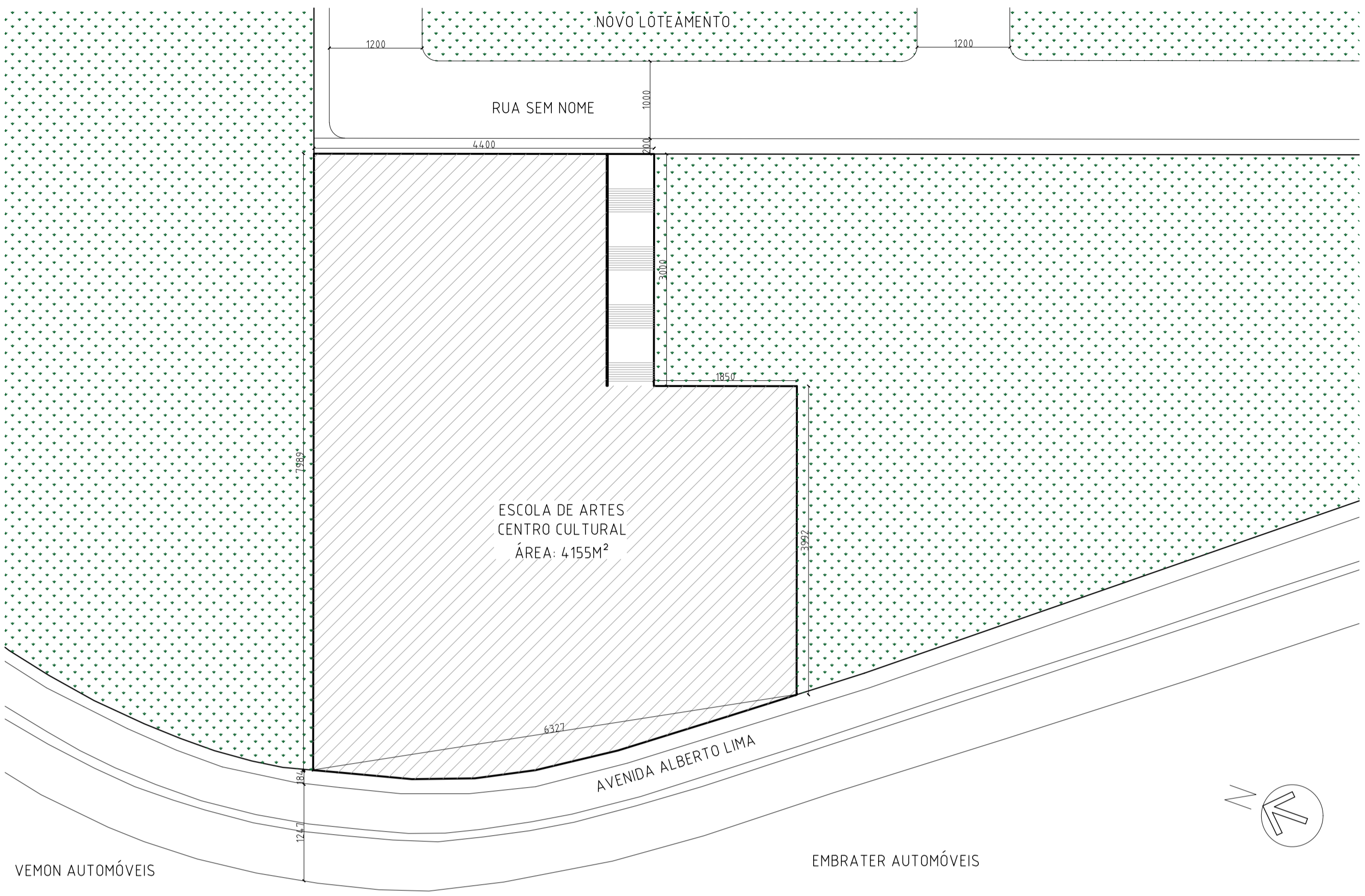
PLANTA DE SITUAÇÃO ESCALA 1/500
