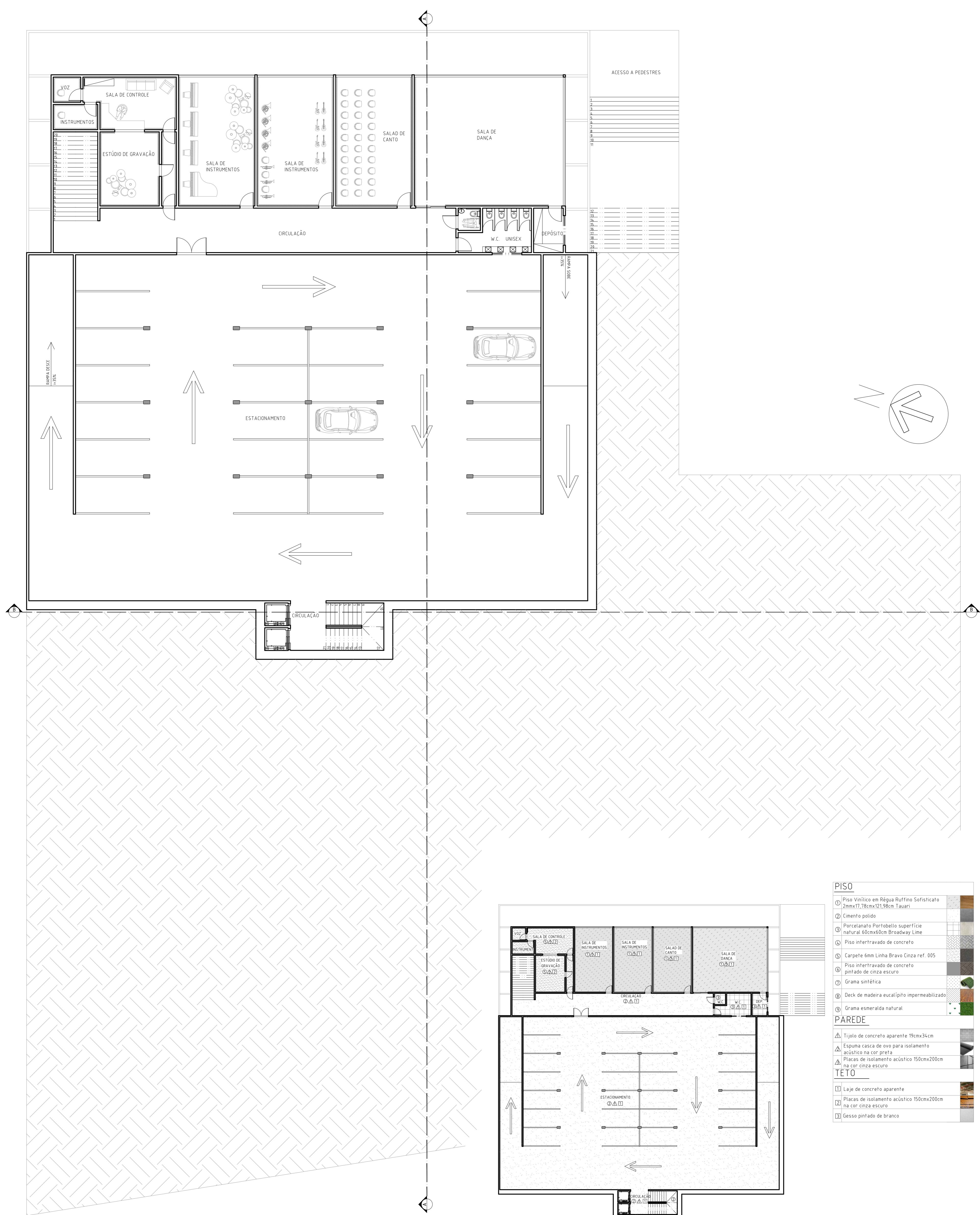
PLANTA LAYOUT 1º PAV. ESCALA 1/250
