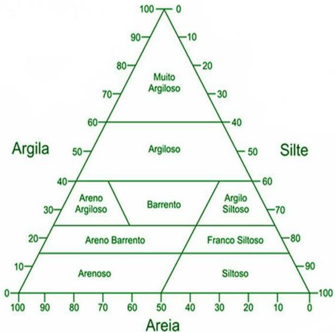
Figura 5 - Classe textural do solo
