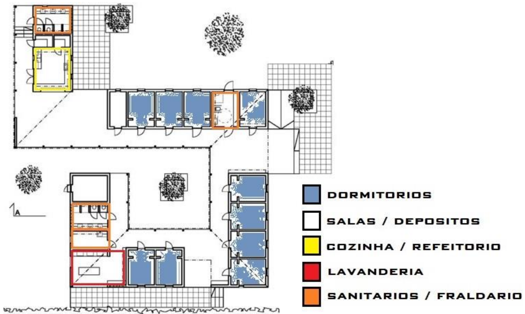
Figura 33 – Planta baixa Casa Albergue KWIECO
