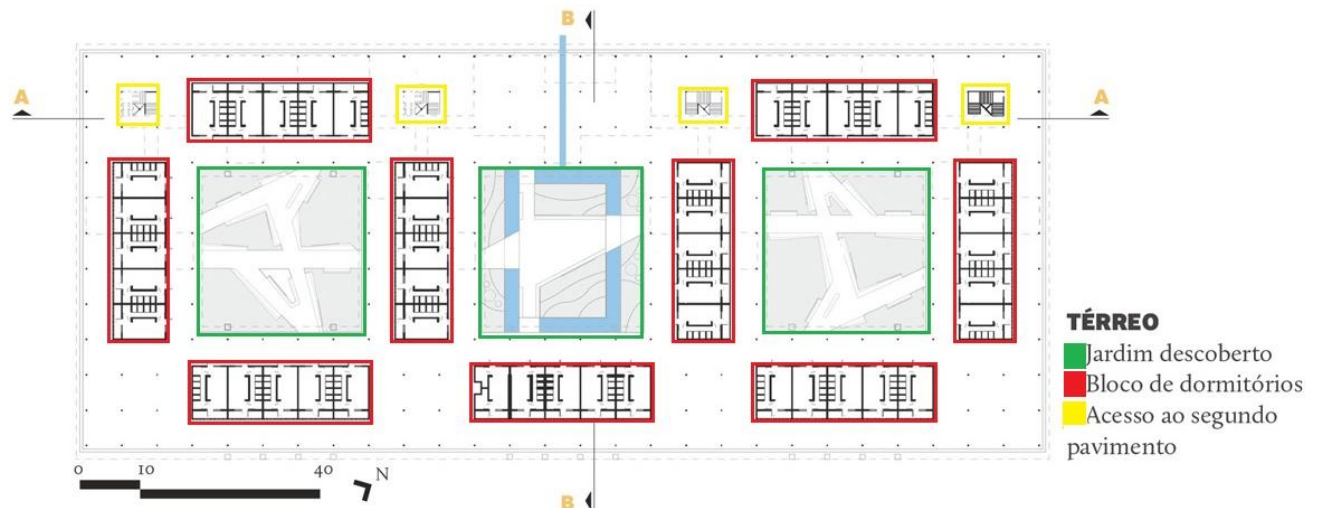
Figura 22 – Planta Baixa térreo -Escola Rural da Fazenda Canuanã
