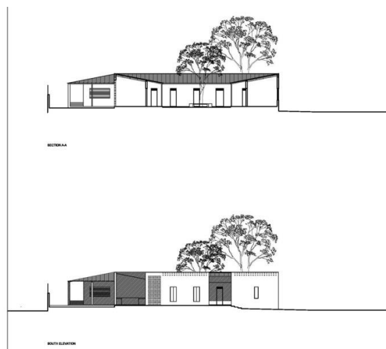
Figura 35 – Cortes Casa Albergue KWIECO
