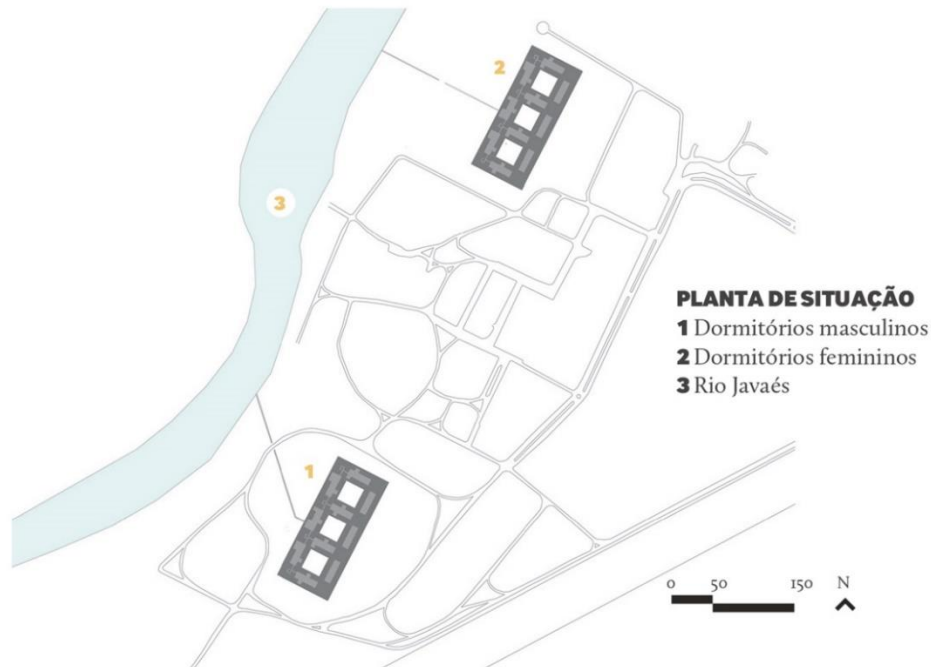
Figura 16 – Planta de Situação
