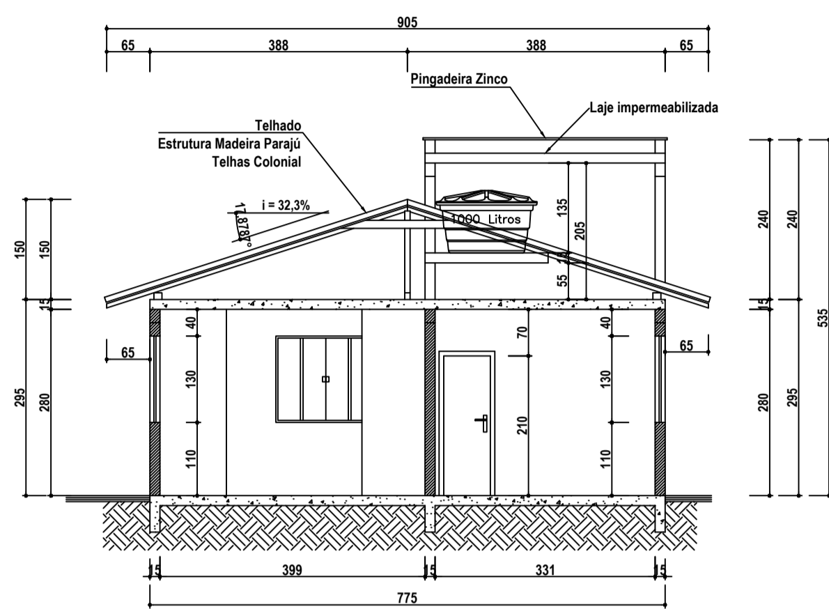
Corte A-A
