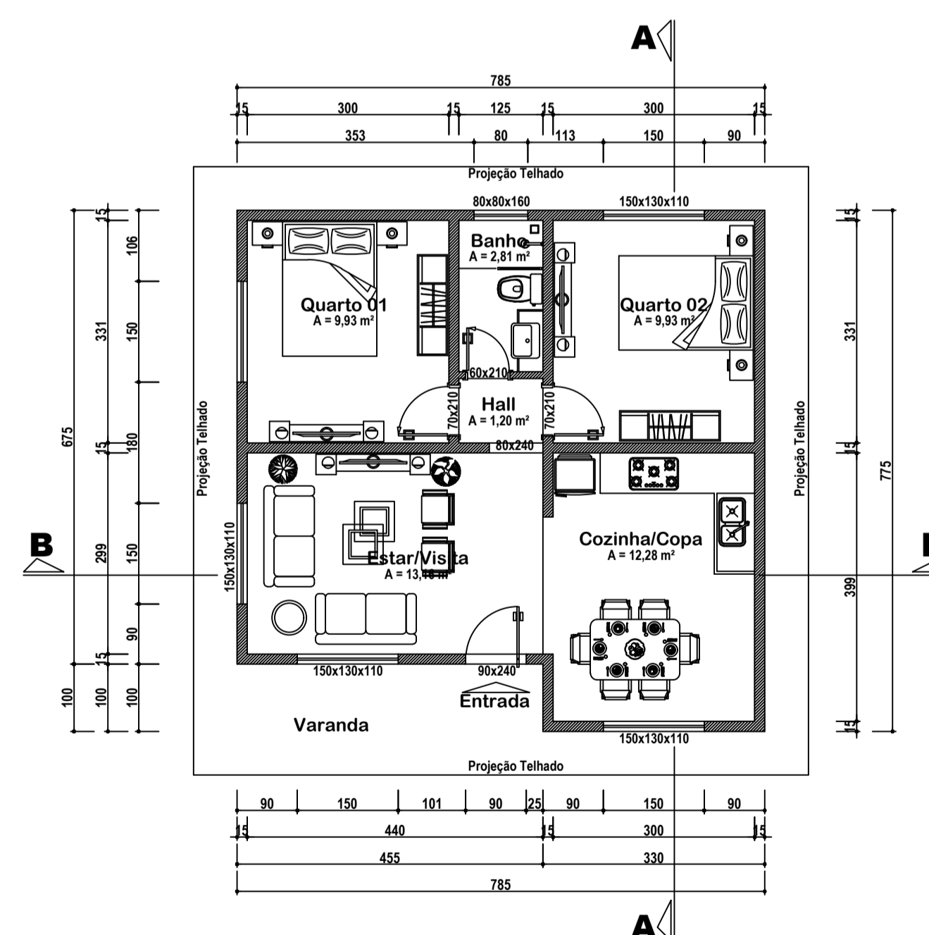
Planta Baixa Térreo
