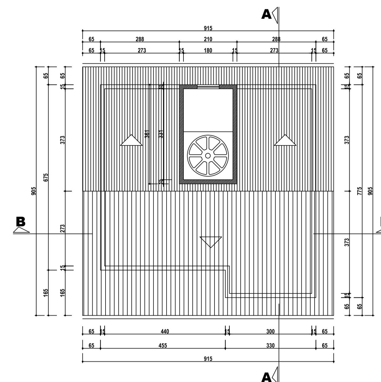
Diagrama Telhado
