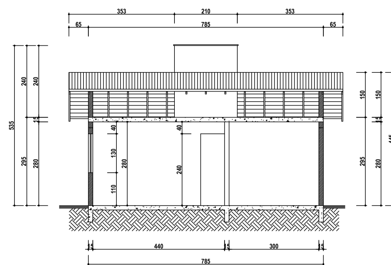
Corte B-B
