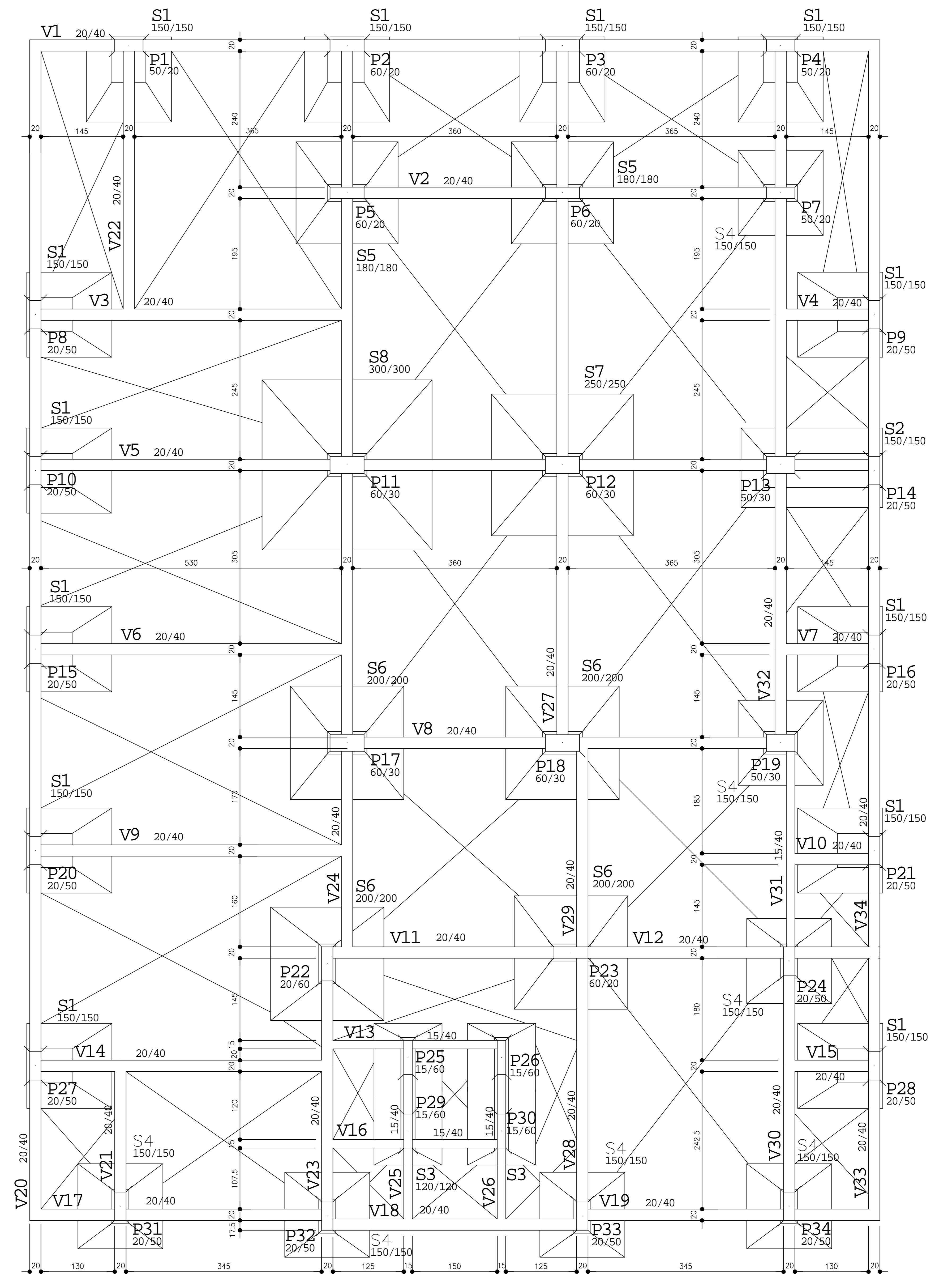
PLANTA DA FORMA DA FUNDAÇÃO
